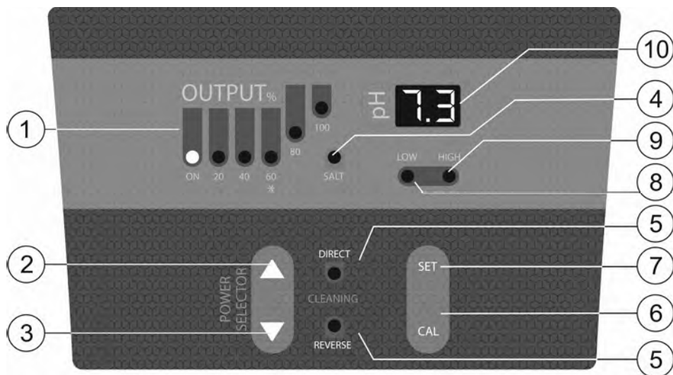
Fig. 15. Panou de control la sistemele MOD. XX-PH
